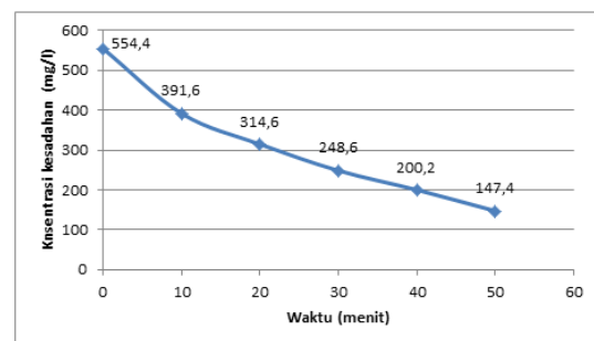
Gambar 2 Kurva penurunan kesadahan pada sumur gali 2
