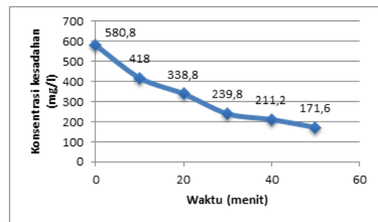
Gambar 1 Kurva penurunan kesadahan pada sumur gali 1
